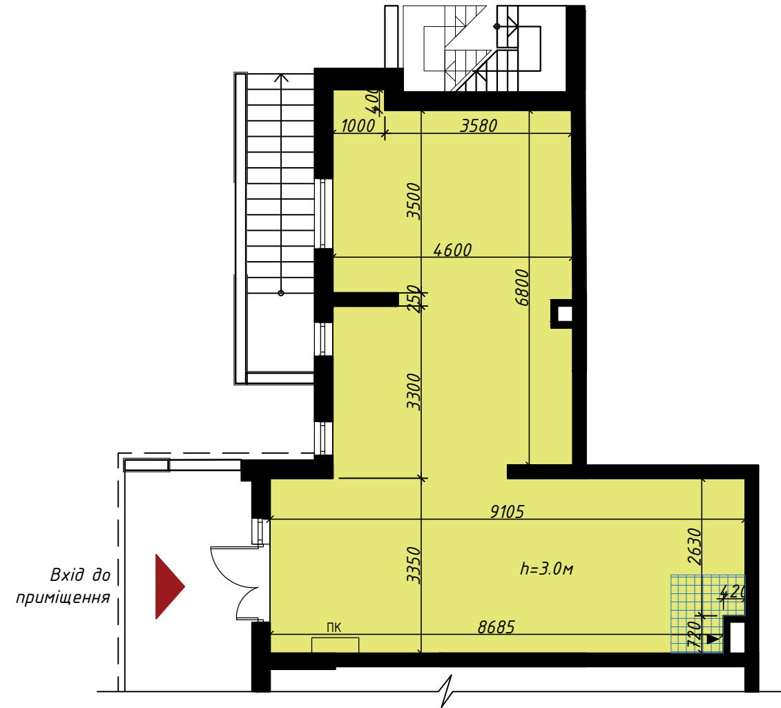
План приміщення з основними розмірами (будівельні розміри, без урахування штукатурки)
