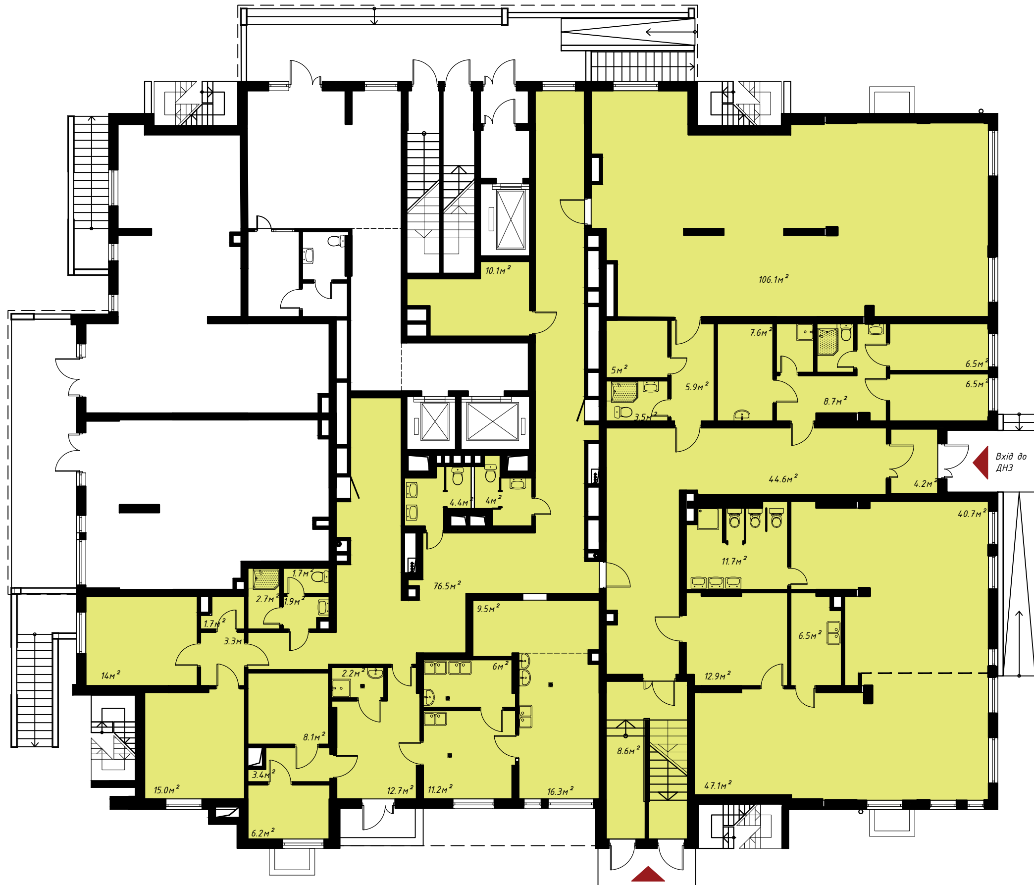
План розташування приміщень ДНЗ 1-го поверху
