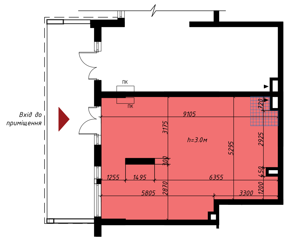
План приміщення з основними розмірами (будівельні розміри, без урахування штукатурки)
